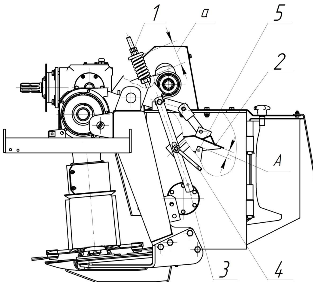
Рисунок 11 – Крепление ножа
