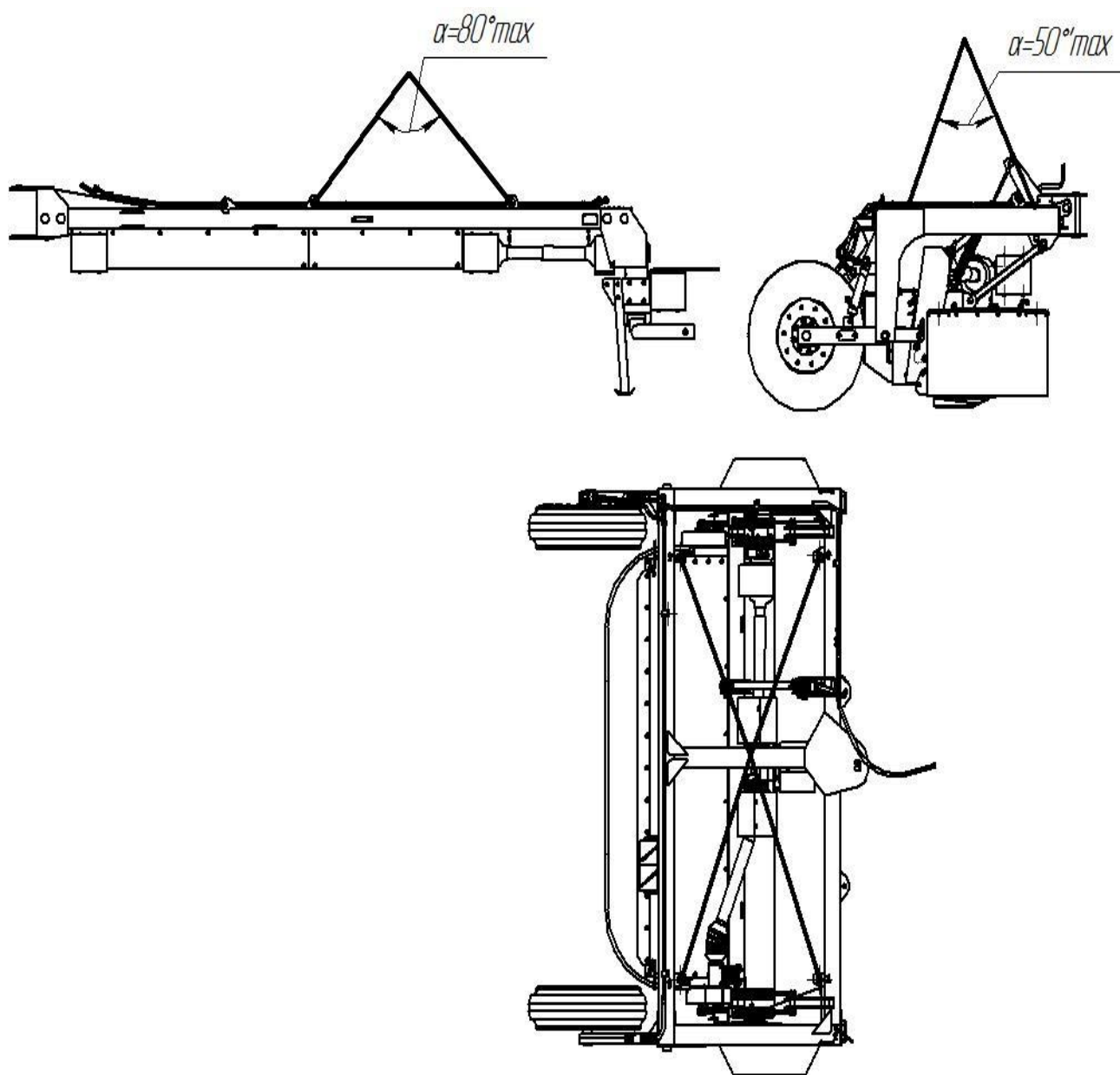
Рисунок 15 – Схема строповки косилки
