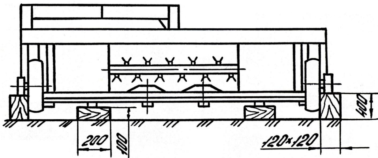
Рисунок 14 – Схема установки косилки на хранение
