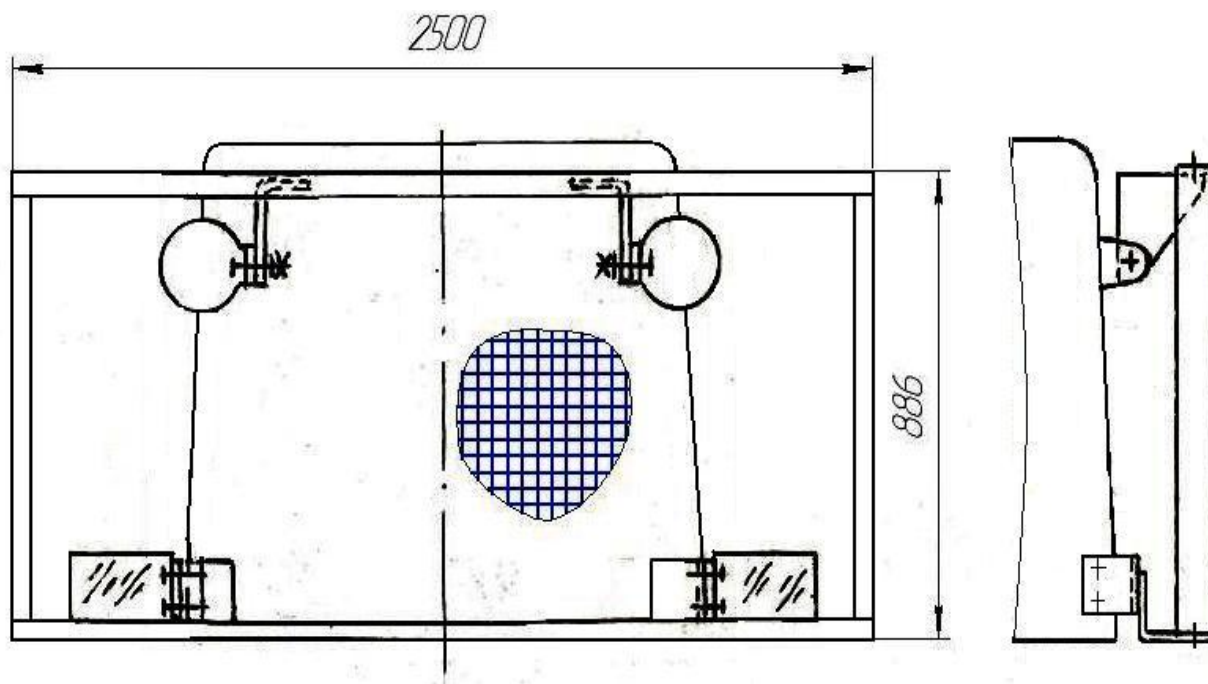
Рисунок 4 – Ограждение кабины трактора
